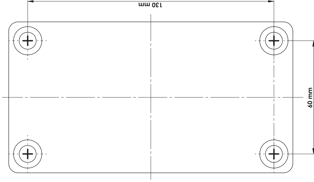
Abbildung A: Bohrschablone Wandhalterung
